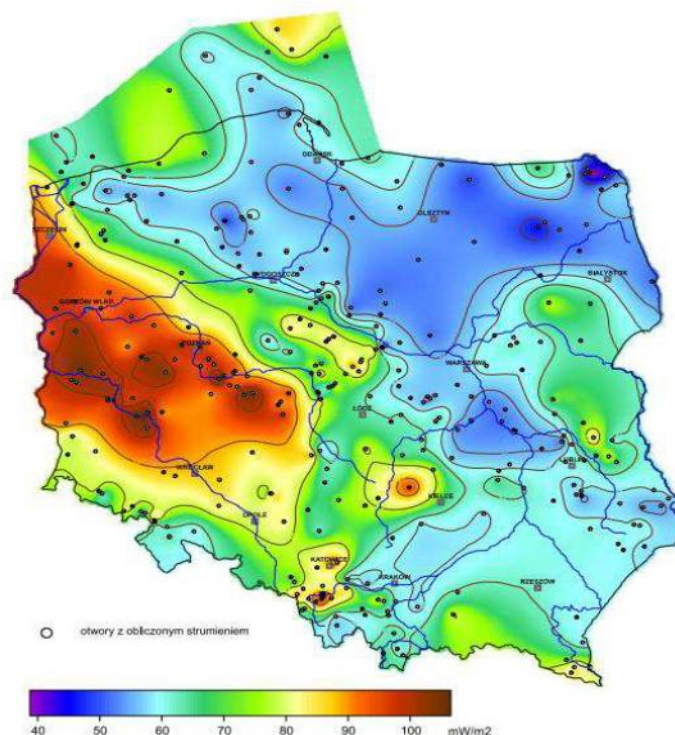
Ryc. 15. Mapa rozkładu gęstości ziemskiego strumienia ciepłego na obszarze Polski Źródło: https://www.mos.gov.pl/ (Szewczyk & Gientka, 2009).
