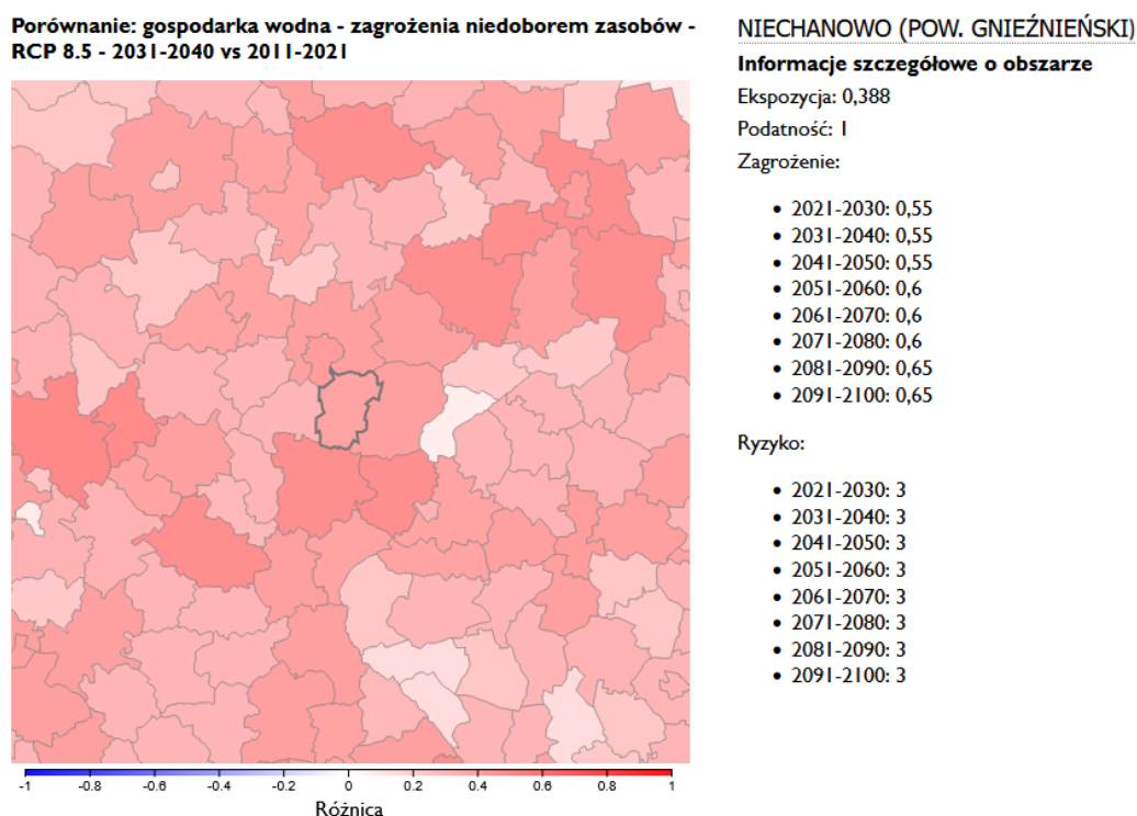
Ryc. 11. Analiza ryzyka w zakresie zagrożenia niedoborem zasobów wodnych w Gminie Niechanowo. Źródło: https://ryzyko.ios.gov.pl/ (dostęp: 19.02.2026).
