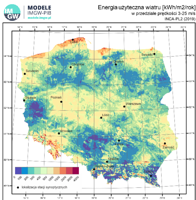
Ryc. 13. Energia użyteczna wiatru na poziomie 10 m n.p.g. w terenie otwartym na obszarze Polski [kWh/m 2 /rok] na podstawie pomiarów z sieci synoptycznej IMGW-PIB (1971-2000).
